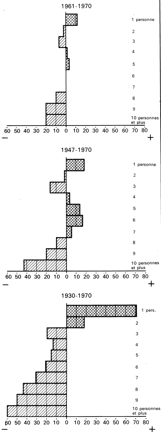
3. — Augmentation ou diminution en % des parts proportionnelles des ménages selon la taille.
