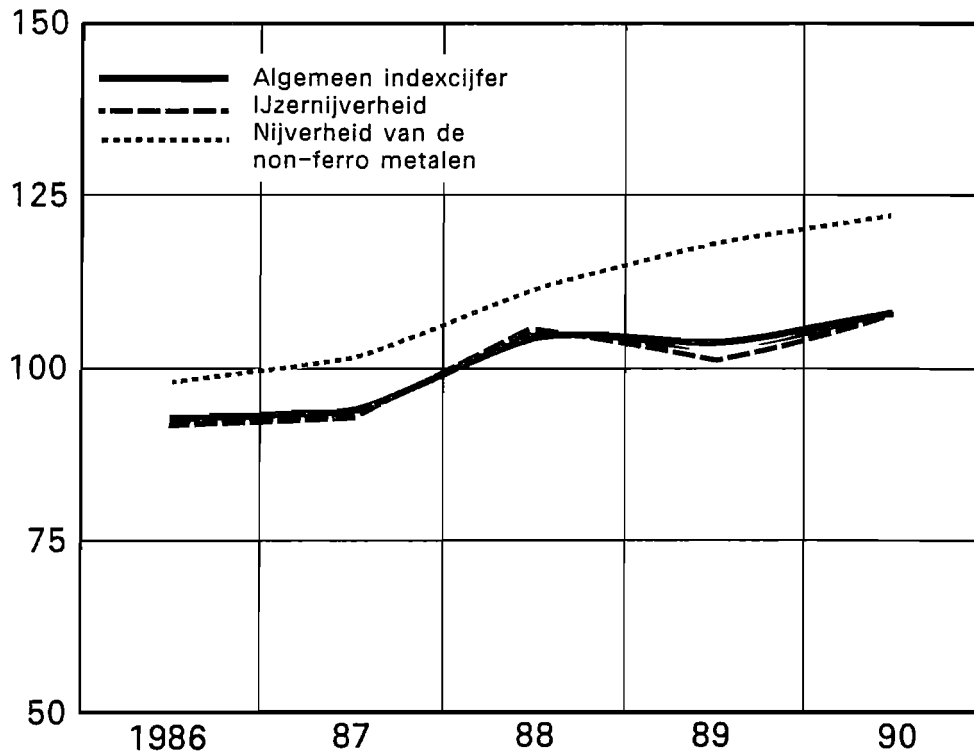
Basis - metaalnijverheid (1985 = 100)
