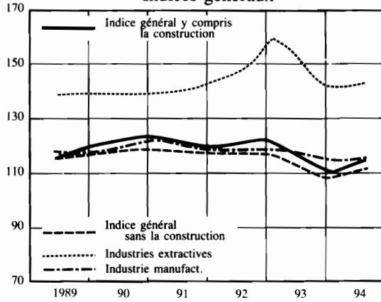
Indices généraux
