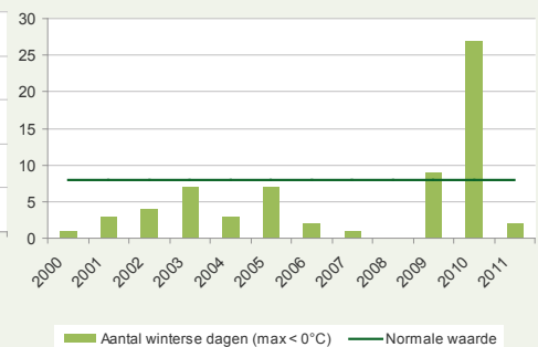
Aantal winterse dagen (max < 0°C)
