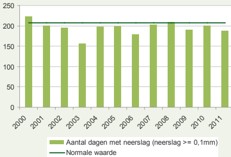
Aantal dagen met neerslag (neerslag >= 0,1mm)
